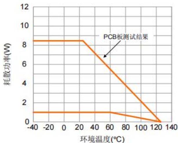
耗散功率 VS 环境温度 (SOT-223)
